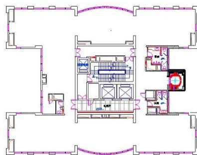
标准层平面图
